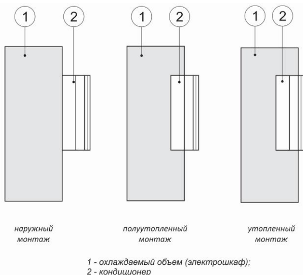
Рис. 2 – Варианты монтажа кондиционера
