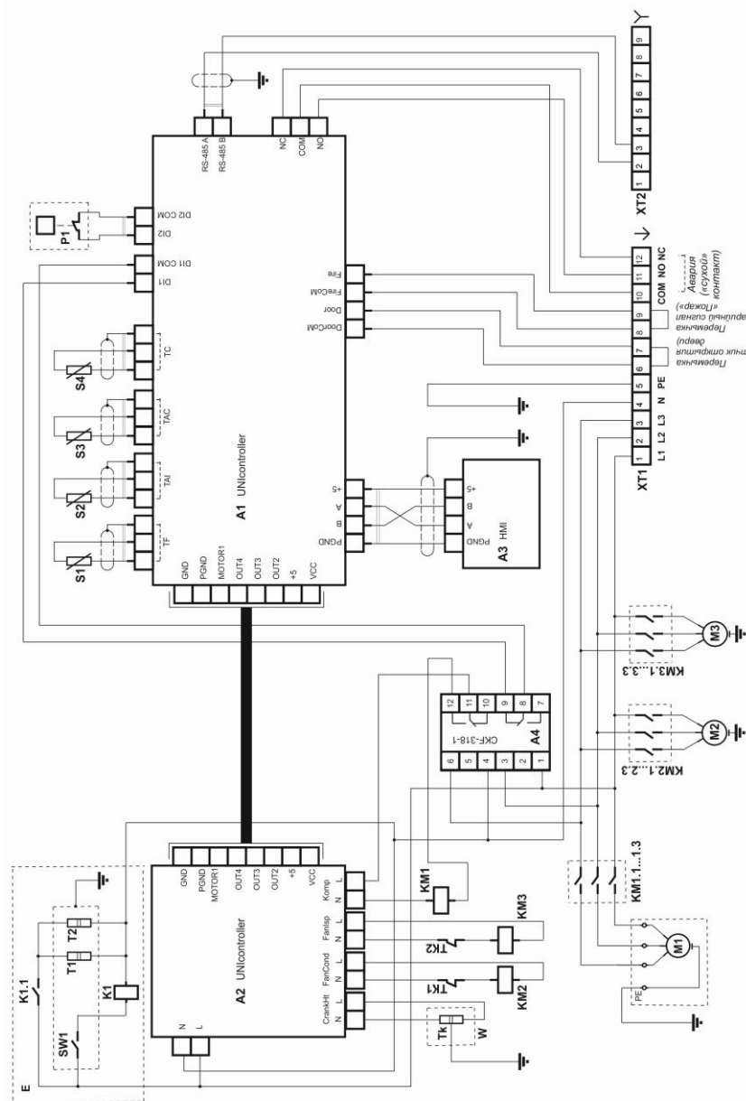
Рис. 4в - Электрическая схема кондиционеров UNISPLIT MHW-560X(3) UNICONTROLLER
