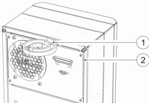
1 – уплотнительная лента; 2 – поверхность стенки, прилегающая к шкафу
